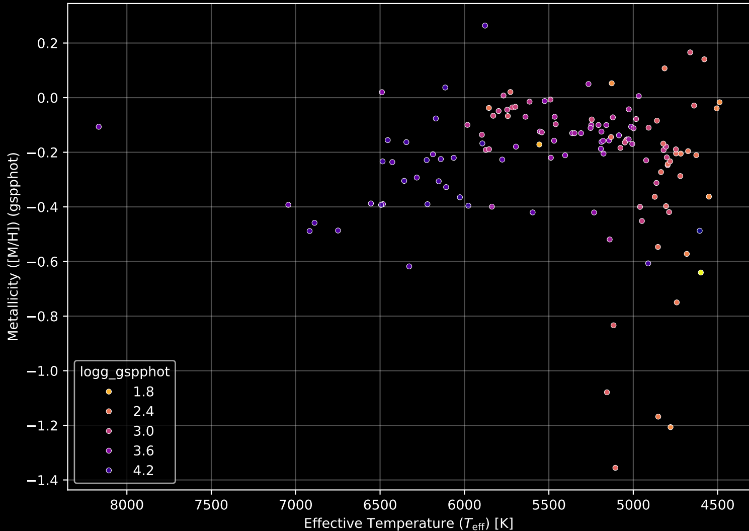
APOGEE DR17 Field: [046+48] Stellar Population Parameters (n= 131)
